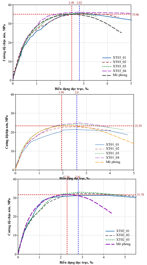
Hình 5.7. So sánh quan hệ ứng suất và biến dạng dọc trục giữa thực nghiệm và mô phỏng (cấp phối XT01, XT02, XT03)
