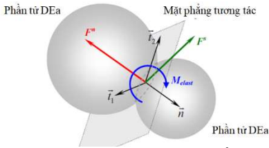
Hình 5.1. Tương tác giữa 2 phần tử và các thành phần lực tương tác
