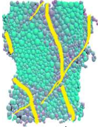
Hình. 5.6. Quan sát vết nứt trên mẫu thí nghiệm số và mẫu thí nghiệm thực nghiệm
