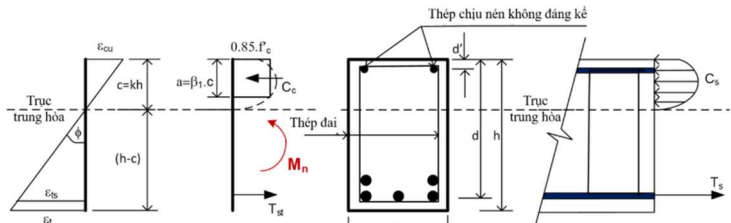
Hình 4.7. Biểu đồ biến dạng và nội lực và lực kéo của thép trong tiết diện thẳng góc với trục dọc của dầm BTCTXT
