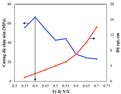
Hình 3.14. Ảnh hưởng của tỷ lệ N/X lên độ sụt và cường độ nén của BTXT ở tuổi 28 ngày, mẫu 100x100x100 mm
