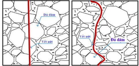
Hình 3.7. Các dạng phá hoại của bê tông dùng cốt liệu là đá tự nhiên
