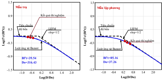
Hình 3.12. Áp dụng luật hiệu ứng kích thước Bazant cho BTXT
