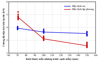
Hình 3.16. Ảnh hưởng của kích thước và hình dạng lên cường độ chịu kéo khi ép chẻ
