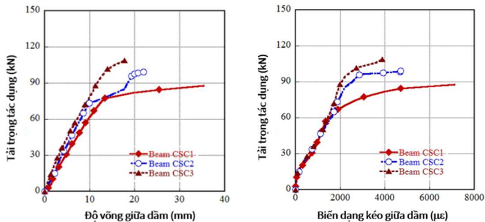
Hình 4.4. Ứng xử uốn của dầm BTCTXT
