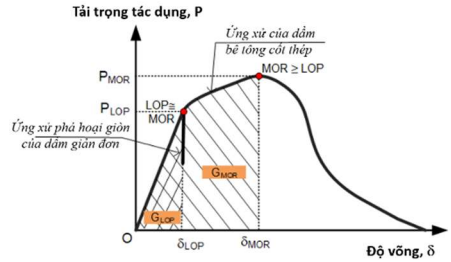
Hình 3.18. Quan hệ giữa tải trọng tác dụng và chuyển vị của BTXT
