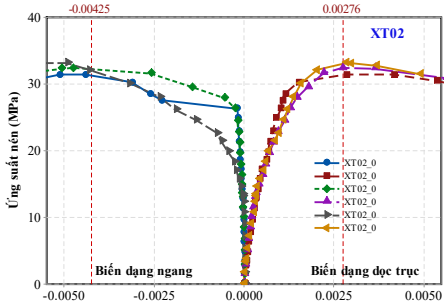
Hình 3.9. Quan hệ giữa ứng suất và biến dạng của 3 loại cấp phối BTXT
