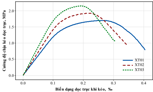
Hình 5.7. Quan hệ giữa ứng suất kéo và biến dạng dọc trục trong thí nghiệm mô phỏng kéo dọc trục mẫu thí nghiệm số XT01, XT02, XT03
