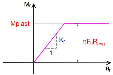
Hình 5.4. Mô men chuyển tiếp giữa các phần tử tương tác [62]
