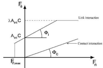
Hình 5.3. Tiêu chuẩn Mohr – Coulomb dùng trong mô hình [62]
