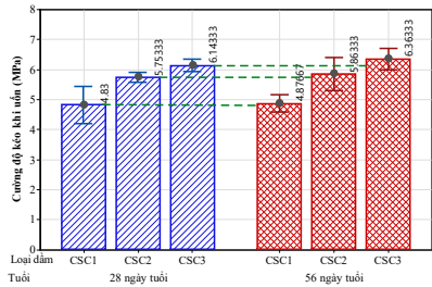
Hình 3.17. f_{cr} ở tuổi 28 và 56 ngày
