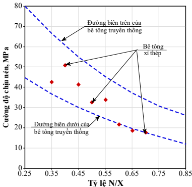
Hình 3.13. Quan hệ giữa cường độ chịu nén và tỷ lệ N/X của BTXT và BTTT, sử dụng mẫu trụ 150x300 mm [92]
