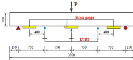
b. Sơ đồ thí nghiệm
