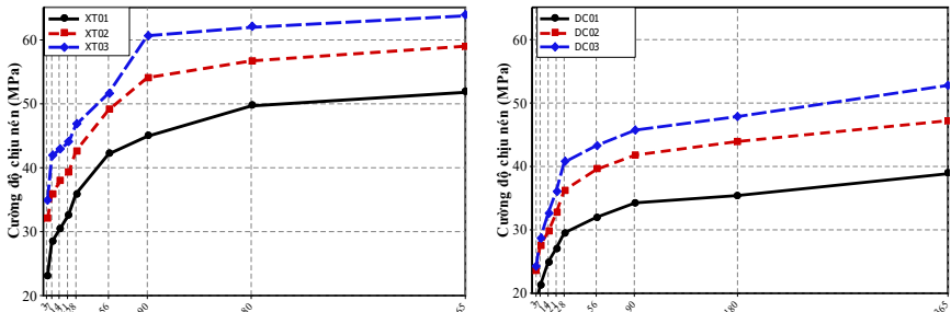
Hình 3.8. Sự phát triển cường độ bê tông theo thời gian
