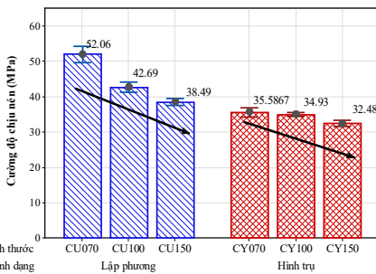
Hình 3.11. Mối quan hệ giữa cường độ chịu nén và kích thước, hình dạng của mẫu
