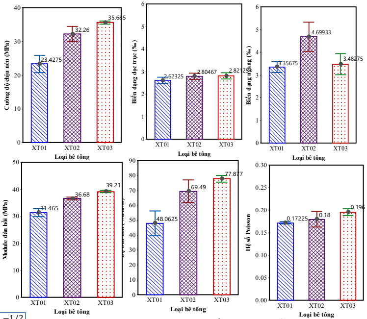
Hình 3.2. So sánh các thông số nén của mẫu BTXT
