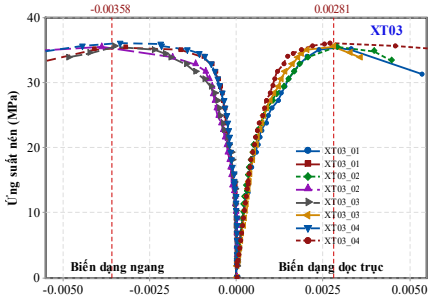
Hình 3.9. Quan hệ giữa ứng suất và biến dạng của 3 loại cấp phối BTXT
