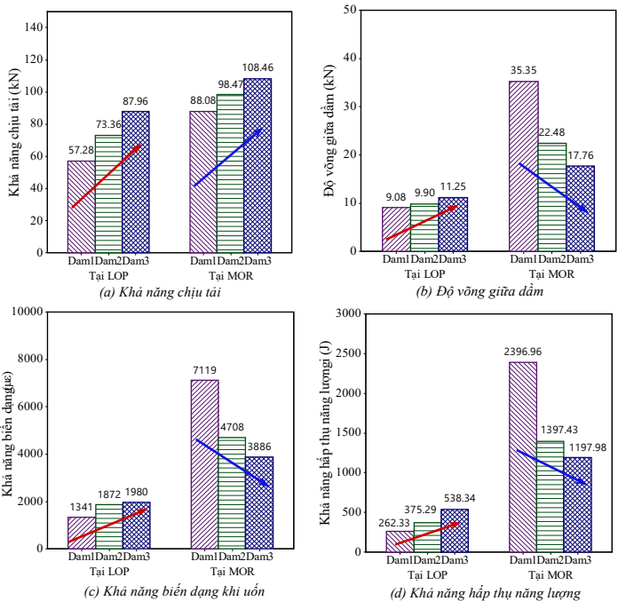
Hình 4.5. So sánh khả năng kháng uốn của 3 dầm BTCTXT
